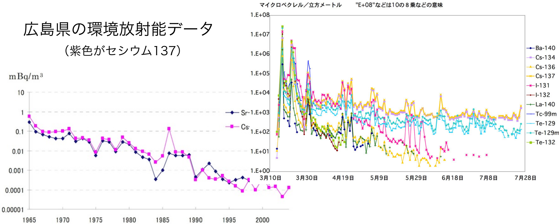
図1 大気浮遊じん中の Sr-90 及び Cs-137 の経年推移
